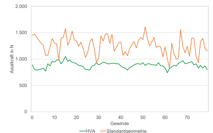
Diagramm: Vergleich des Axialkraftverlaufs
